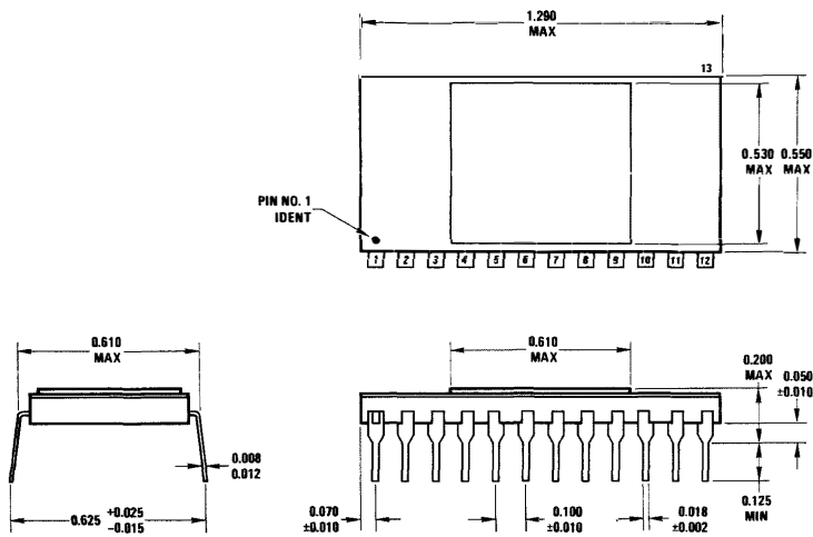
Cavity Dual-In-Line Package (D)
